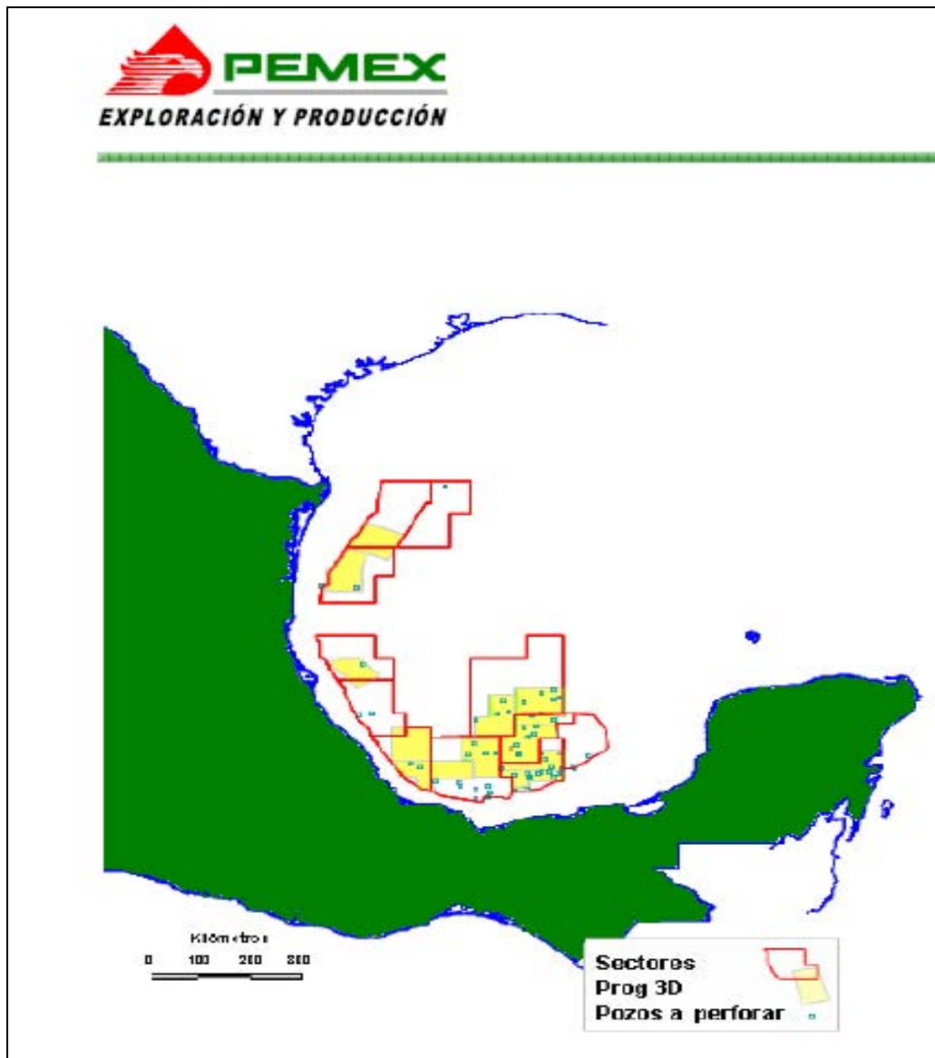
MAPA 3- DOCE AREAS DEL GOLFO DE MEXICO CON PROGRAMAS DE PERFORACIONES PROFUNDAS
