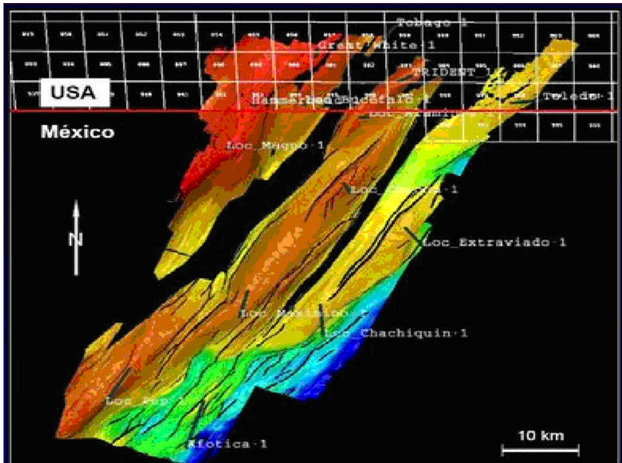
MAPA 4- PRIMER DISEÑO DE LOS NUEVOS BLOQUES EN LA PARTE MEXICANA DEL GOLFO DE MEXICO
