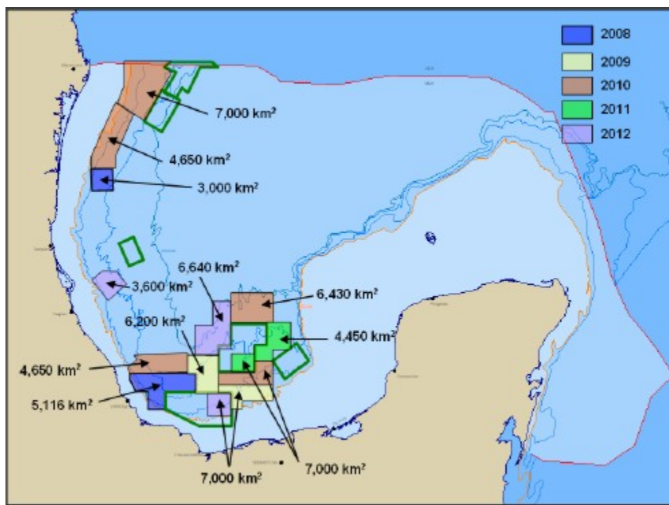
Estudios de sismica 3D realizados por Pemex en el Golfo de México.
