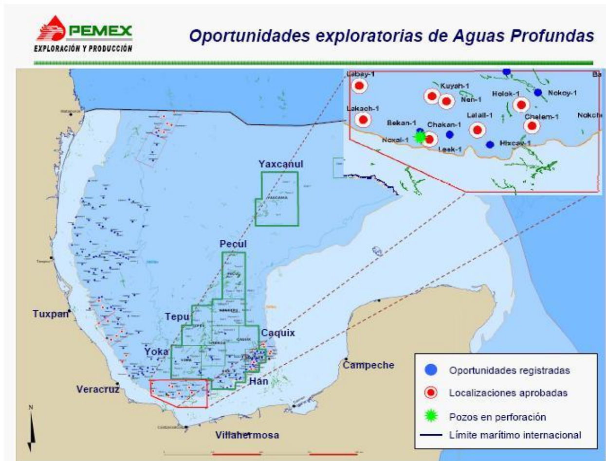
MAPA 2. LAS CHAPOPOTERAS MARINAS
